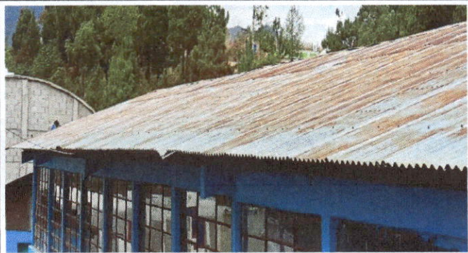
Foto1: Lámina en mal estado, del módulo 1 de aulas. Con 381 M2.
